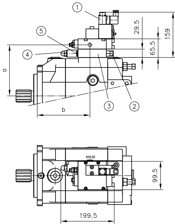
Coding Lfe
