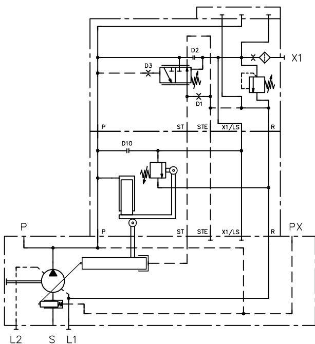
Coding LSPL
