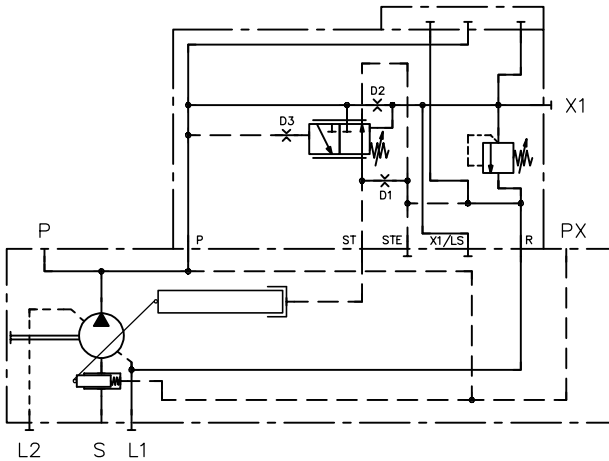
Coding PL
