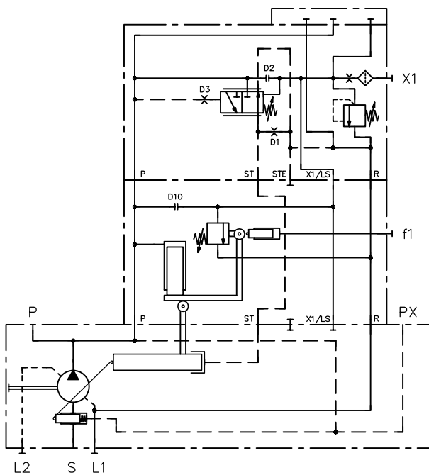
Coding LSPLf1
