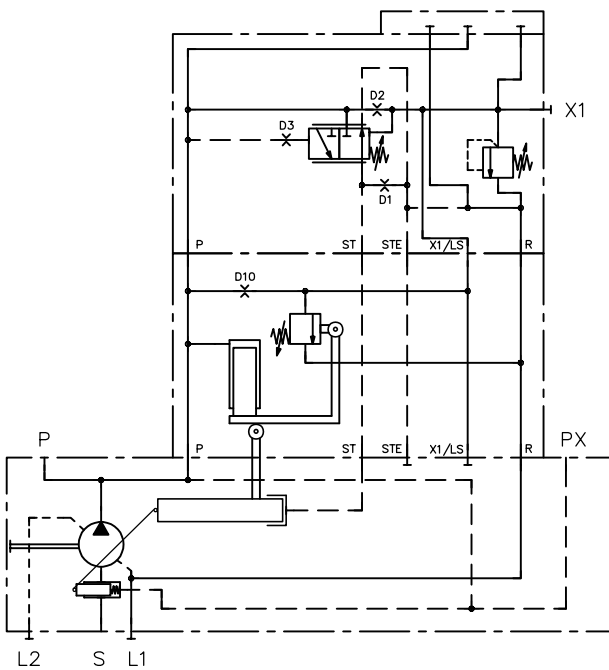
Coding PL
